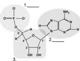
Рисунок 2. Составляющие компоненты нуклеотида
