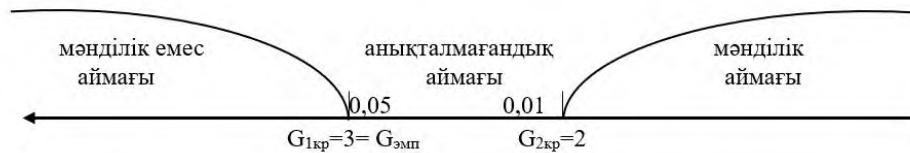
Сурет 1 – G_{эмп} эмпирикалық мәнінің анықталу аймағы
